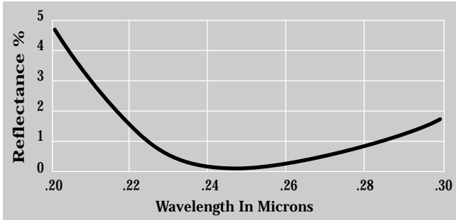
V-coat 248 nm
