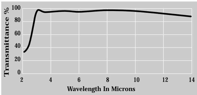
BBAR Si 3-5 um
