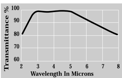
BBAR Si 3-5 um
