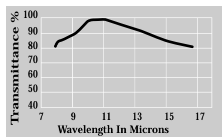
NBAR ZnSe 10.6 um
