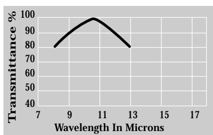
NBAR Ge 10.6 um
