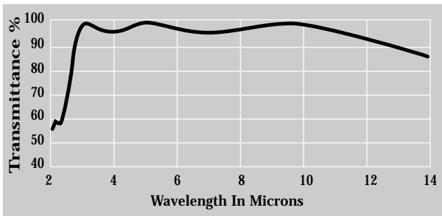
BBAR ZnSe 3-12 um
