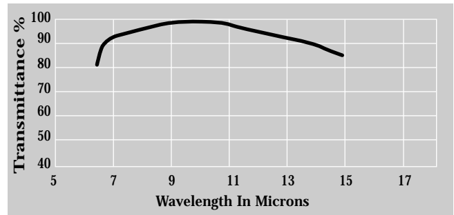
NBAR Ge 10.6 um
