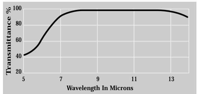
BBAR ZnSe 8-12 um
